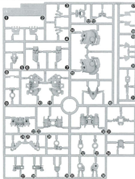
Aパーツ(グレー) (PS) A Parts (Gray)
